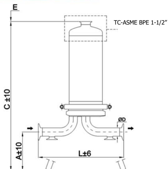
Dimensioni nominali mm
